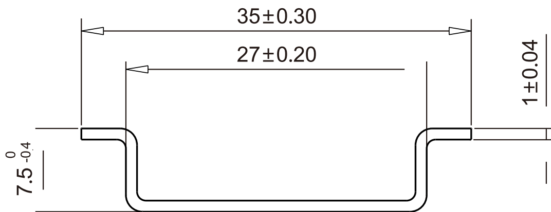
图 2 安装轨尺寸
